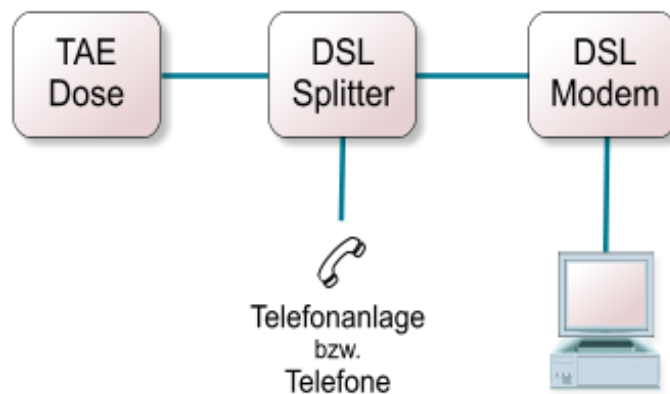
Verkabelung mit einem externen Modem
